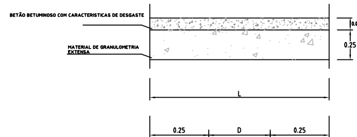
PORMENOR A ESTRUTURA A REPOR TMD = 3.500 VEICULOS DIA
